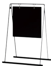
2768 K 360×360 外寸法 W500×H675×D345
